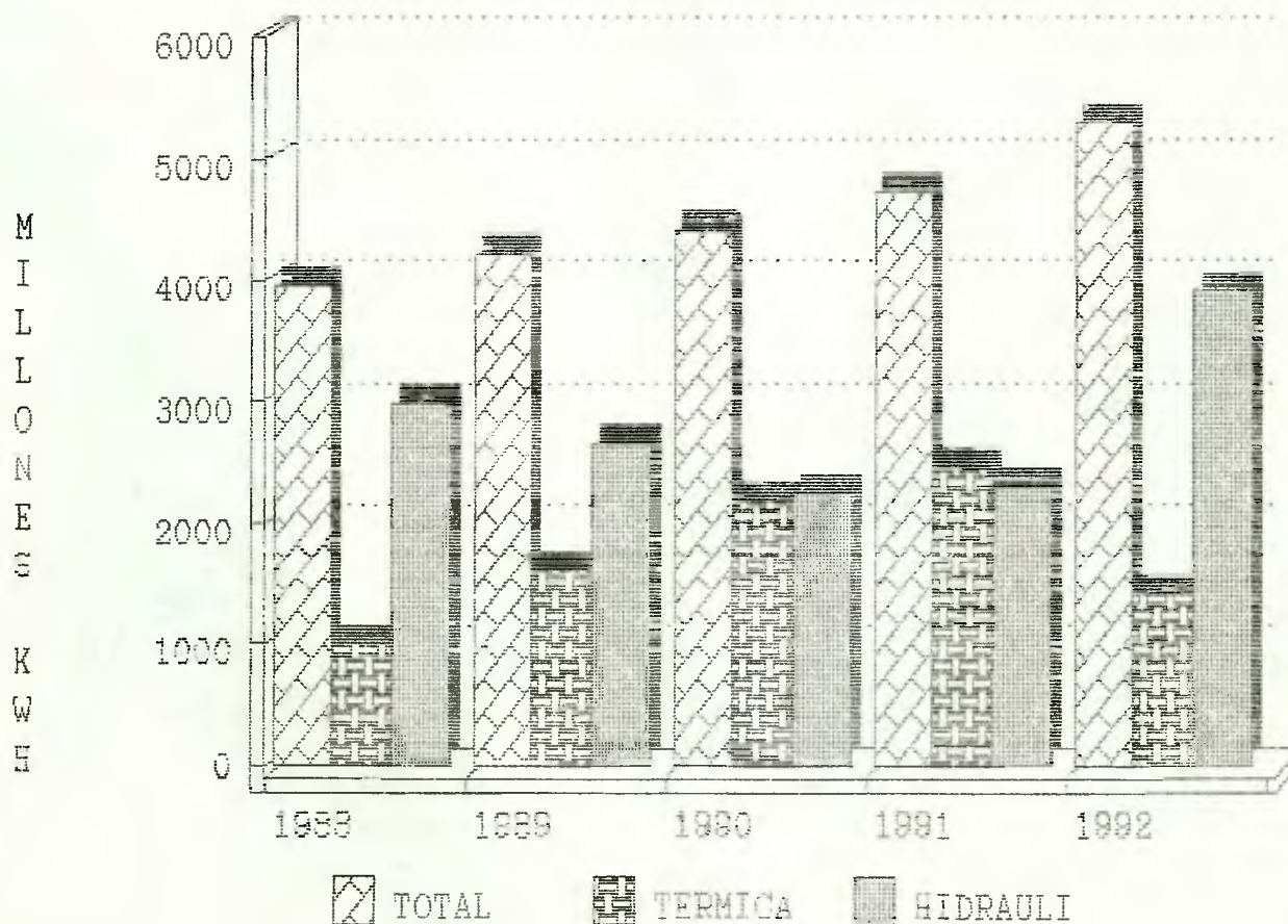
GENERACION DE ENERGIA ELECTRICA ENERO - MARZO 1988 - 92
