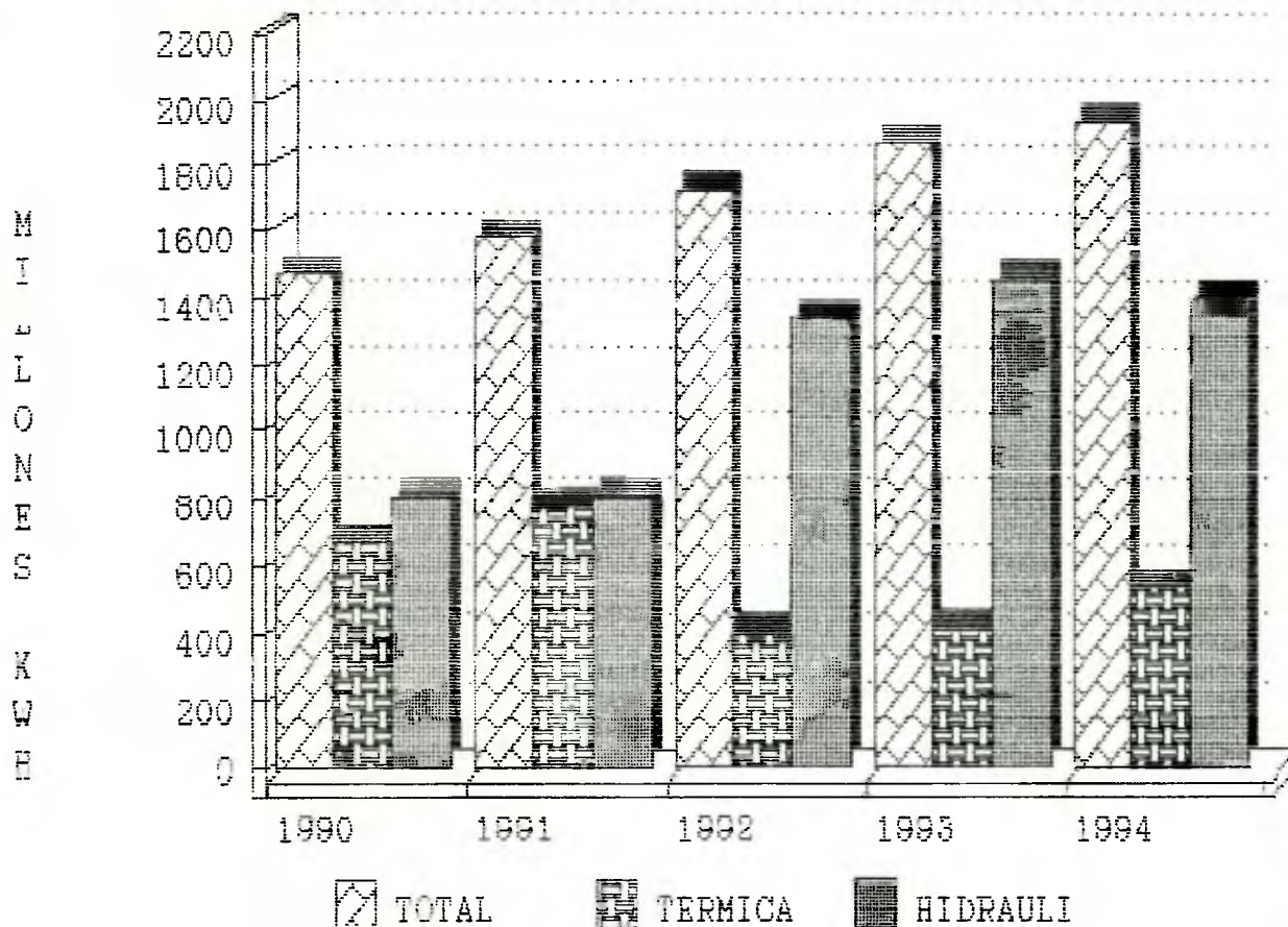
GENERACION DE ENERGIA ELECTRICA ENERO 1990 - 94
