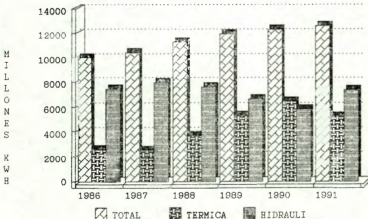
GENERACION DE ENERGIA ELECTRICA ENERO - AGOSTO 1986 - 91
