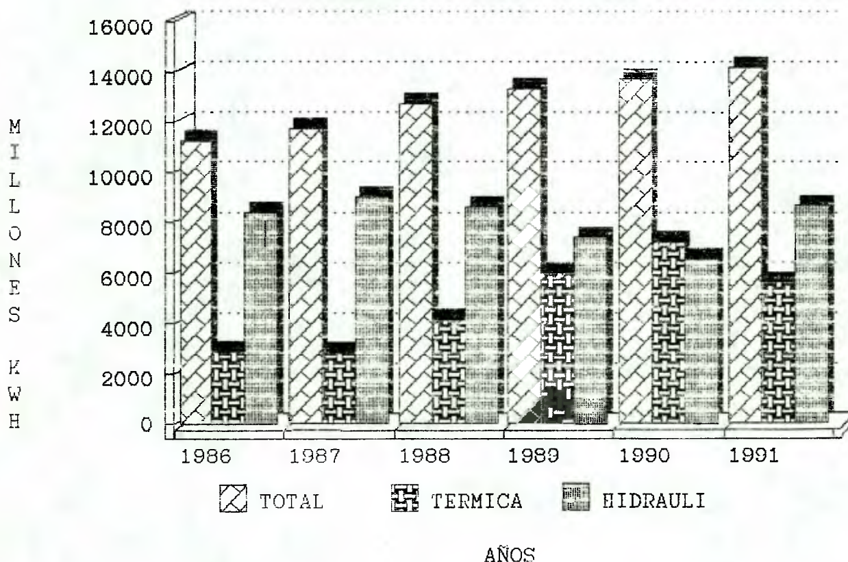
GENERACION DE ENERGIA ELECTRICA ENERO - SEPTIEMBRE 1986 - 91
